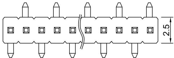
TYPE-A(正脚位)
