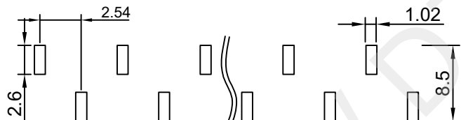
P.C.B LAYOUT
